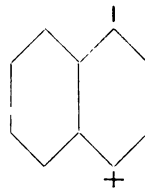
\alpha Säure. Neville u. Winther. Ber. 13. 1949.
